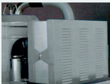
Filtro absoluto de aire de salida: área de filtro de 170,000cm²
